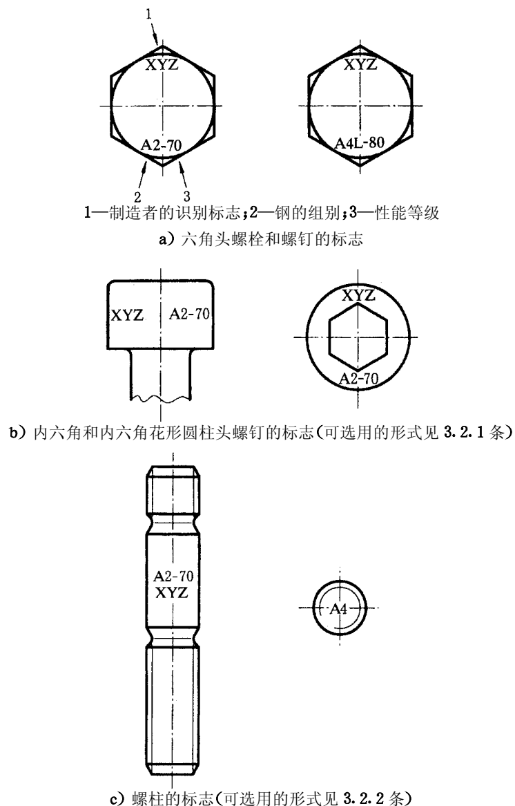
图 2 螺栓、螺钉和螺柱的标志
