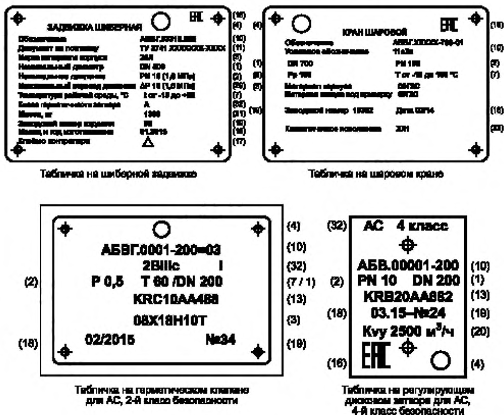
Рисунок Г.5 — Примеры расположения маркировки на табличке
