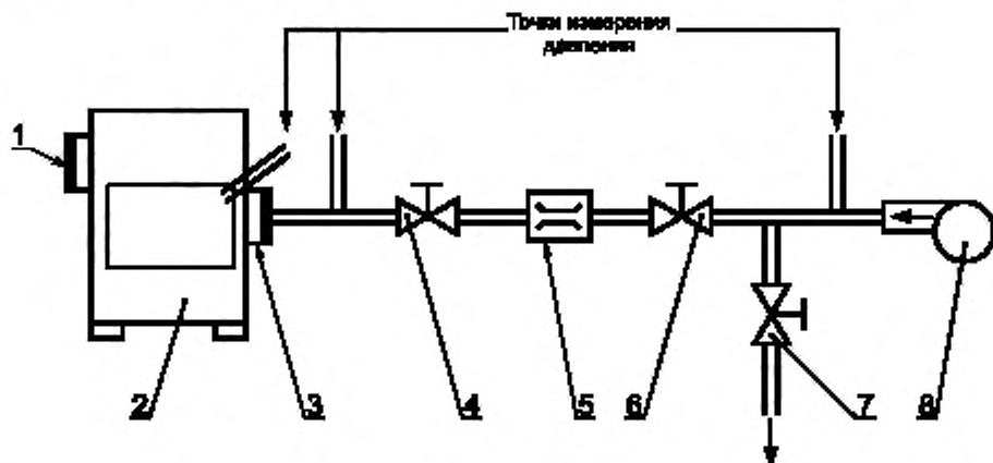
1 — патрубок входящих газов; 2 — испытуемый котел; 3 — амбразура горелки; 4 — регулирующий орган 1; 5 — измеритель расхода; 6 — регулирующий орган 2; 7 — регулирующий орган 3; 8 — вентилятор
