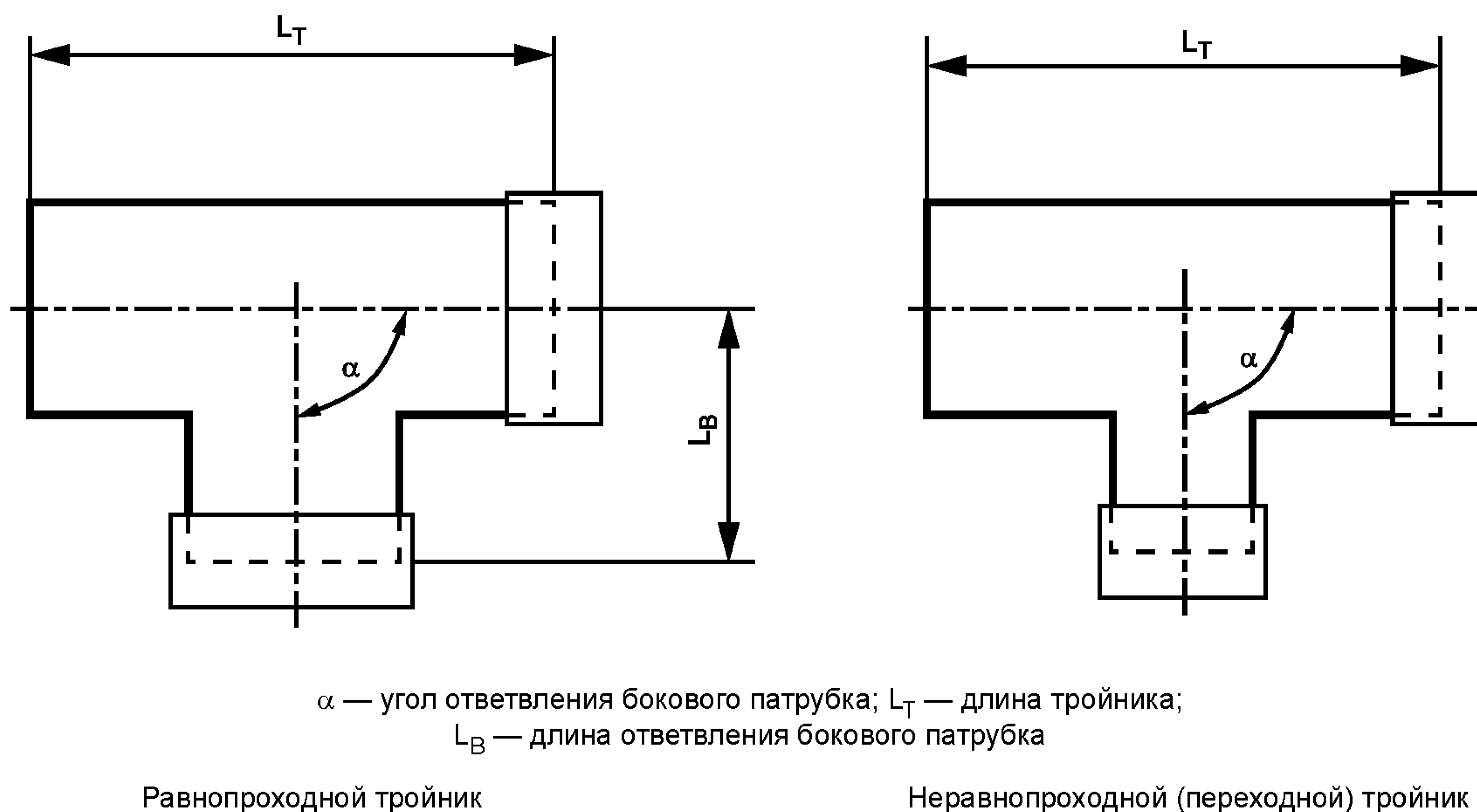
Рисунок 7 — Тройники
