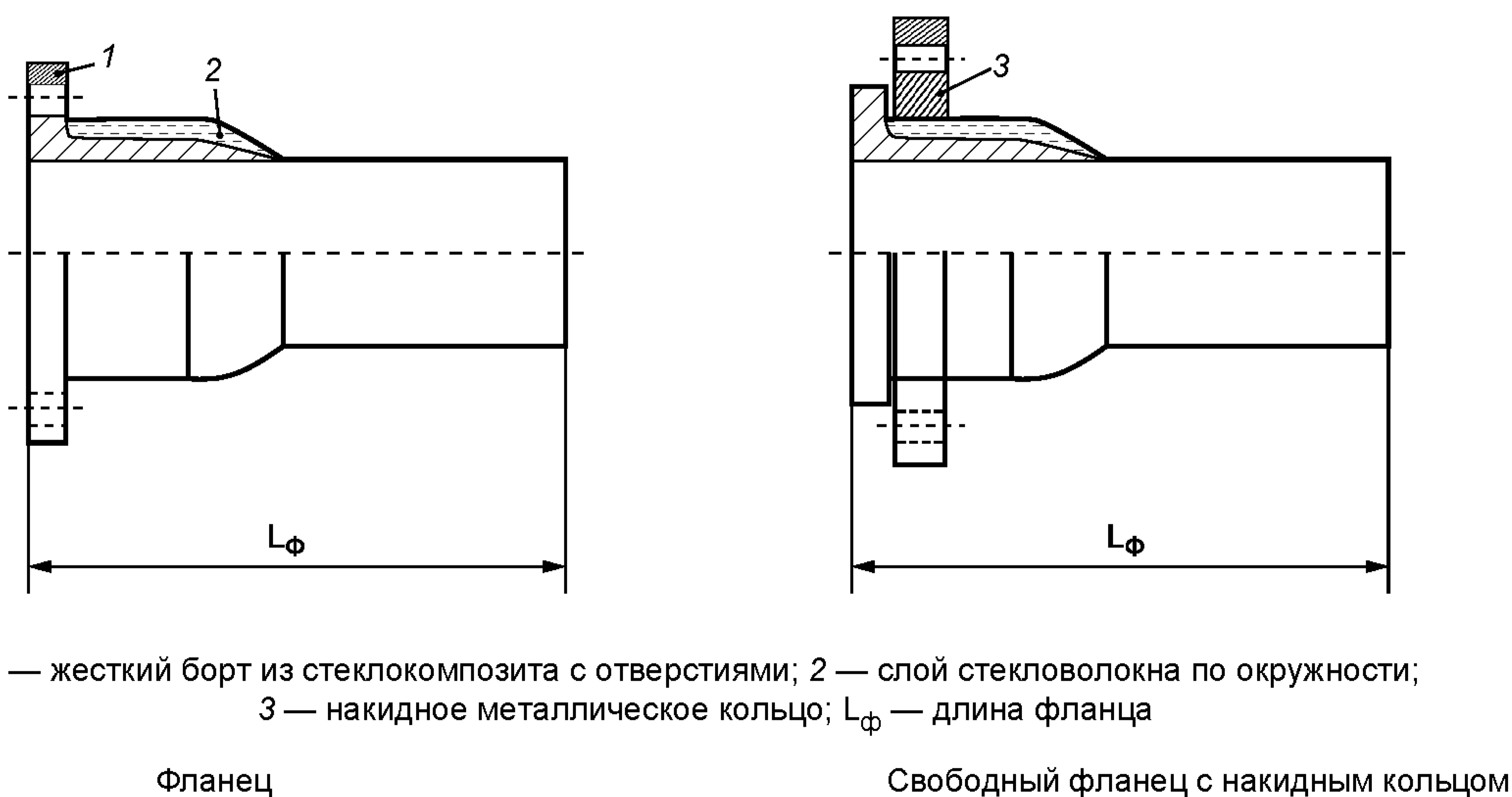
Рисунок 8 — Фланцы
