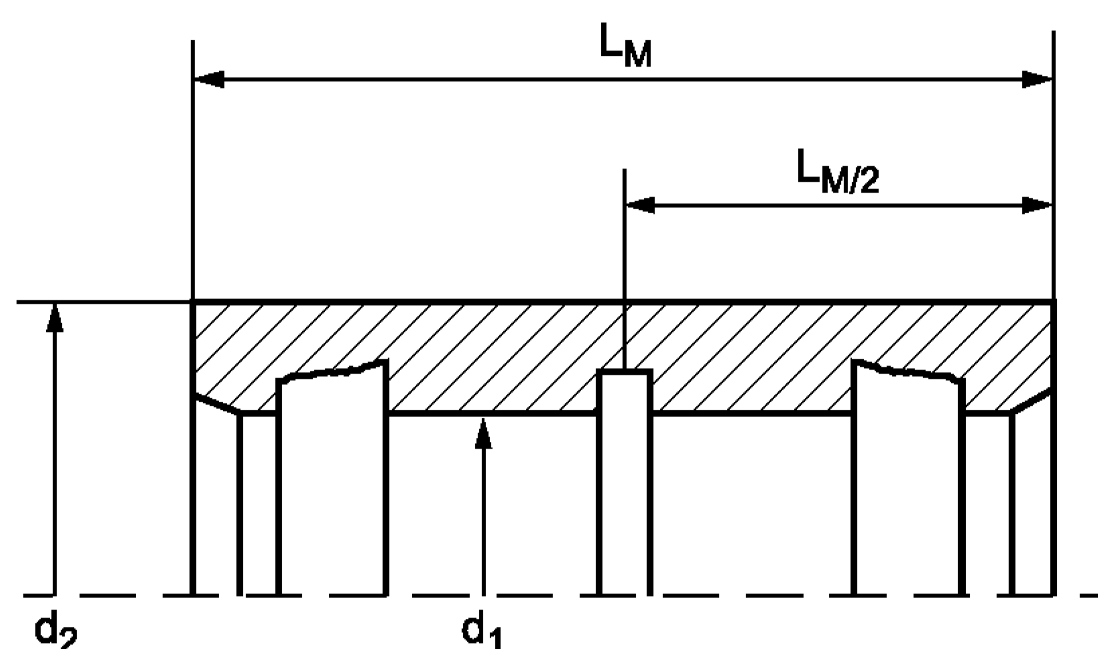
d_1 — внутренний диаметр муфты; d_2 — наружный диаметр муфты; L_M — длина муфты
