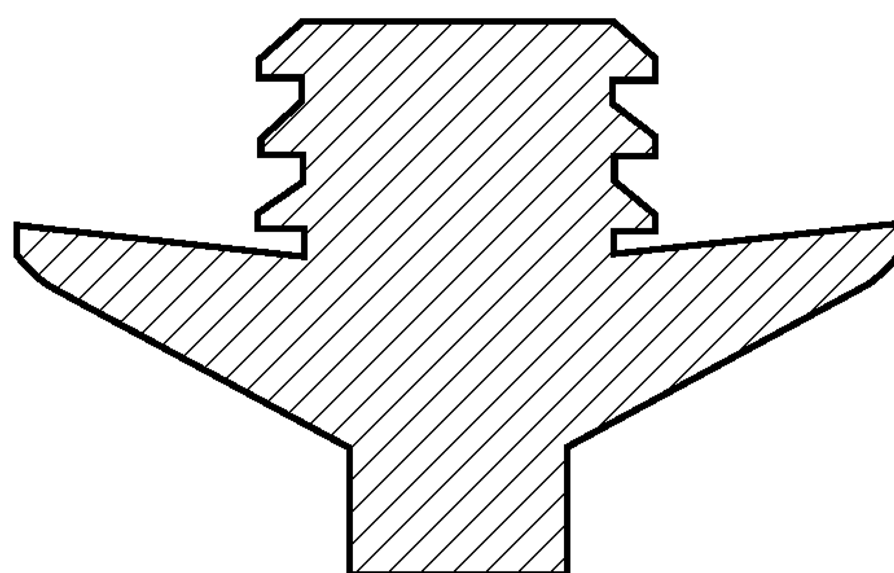
Рисунок 4 — Форма поперечного сечения центрального ограничителя
