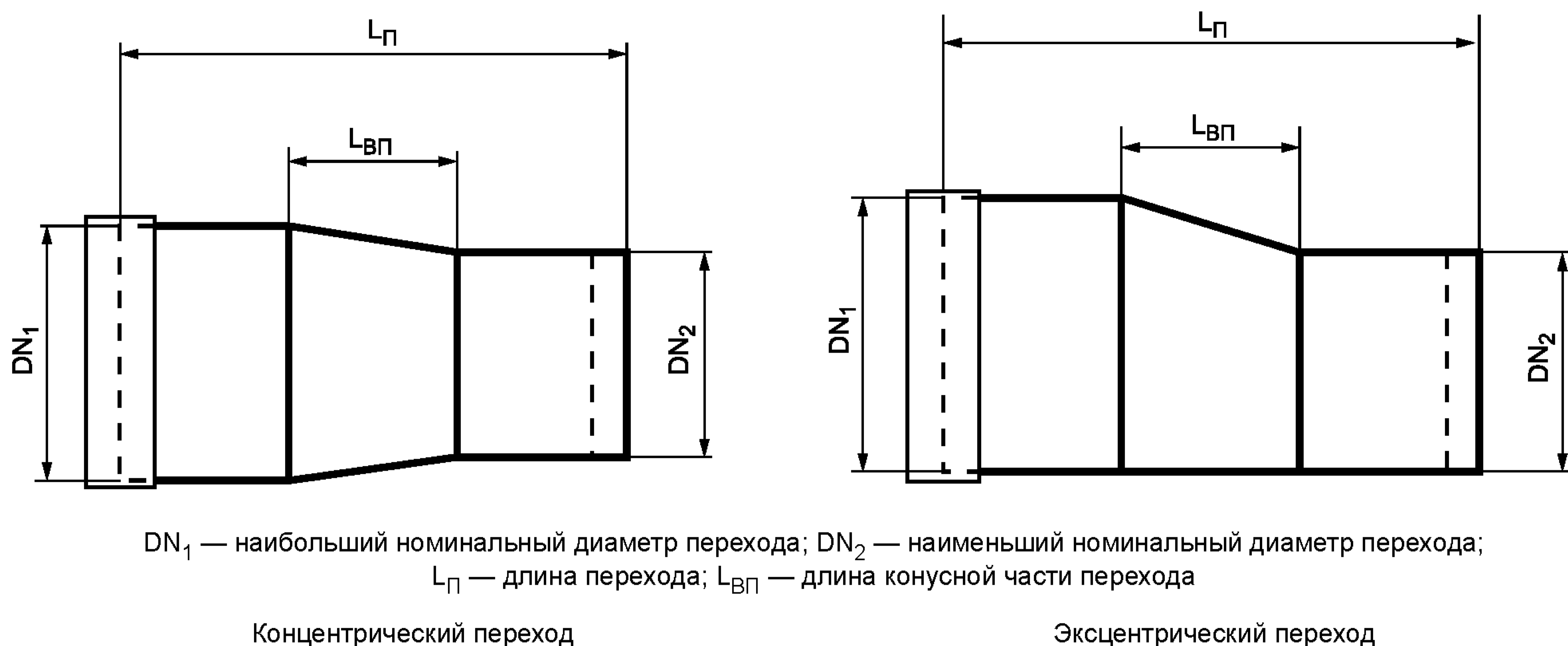
Рисунок 6 — Переходы
