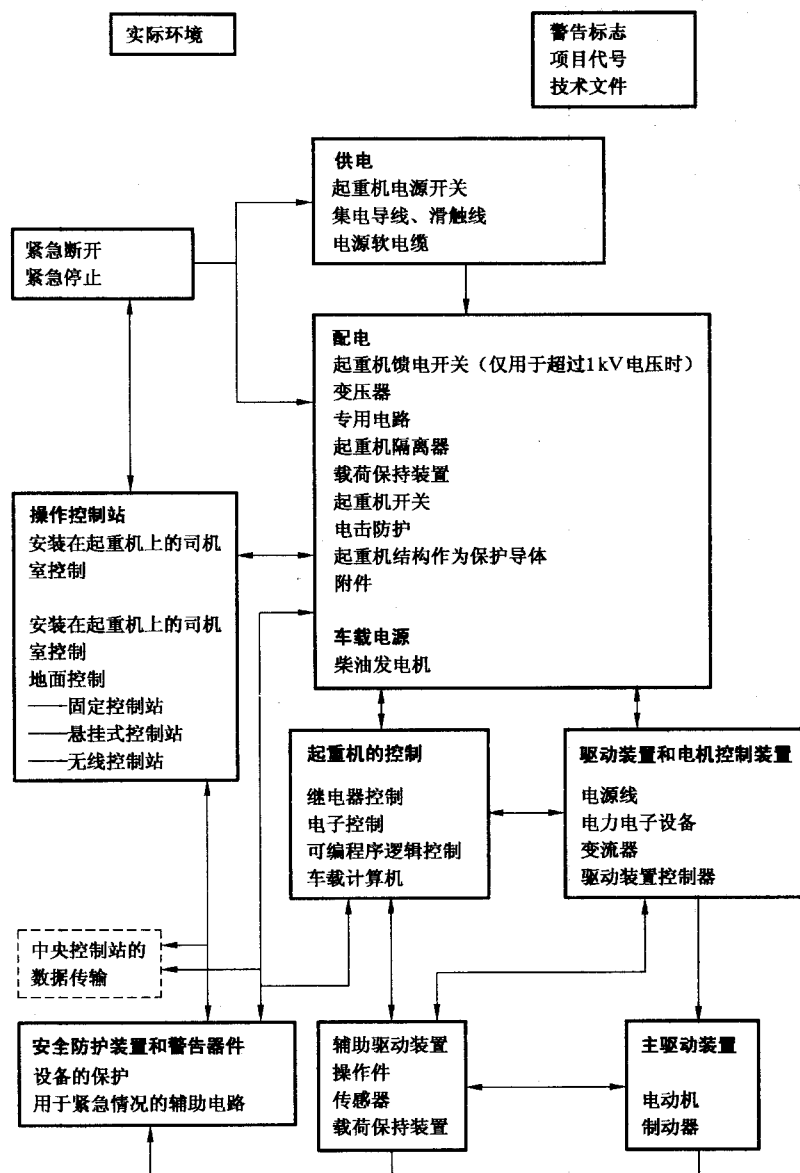
图 2 典型起重机及其相关电气设备的框图
