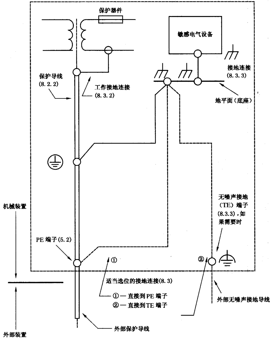
图 4 起重机械电气设备等电位连接示例
