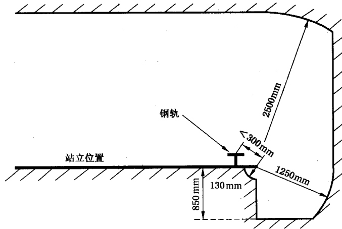
a) 起升装置钢轨中央至主梁边缘距离小于 300 mm 情况下伸臂范围的界限
