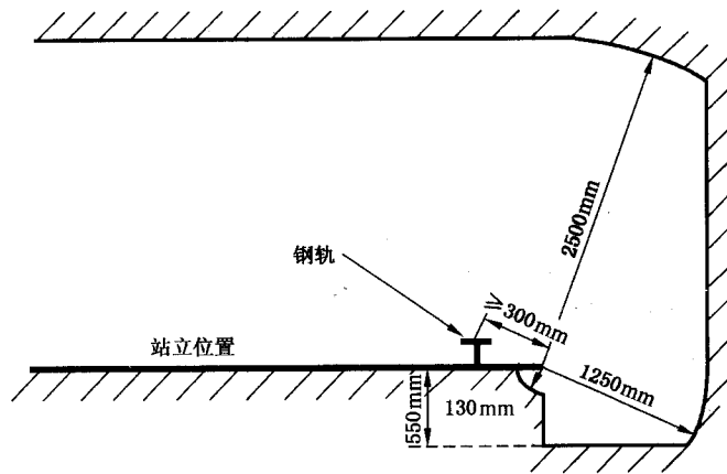
b) 起升装置钢轨中央至主梁边缘距离不小于 300 mm 情况下伸臂范围的界限
