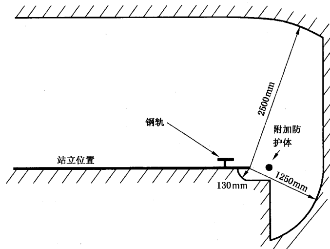
c) 采用附加阻挡物情况下伸臂范围的界限
